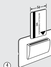
④ Una vez reensamblado el interruptor se podrá accionar con la tarjeta estandar del hotel.
