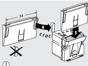
③ Romper las prerrupturas de la sotoplaça y reensamblarla con el interruptor.
