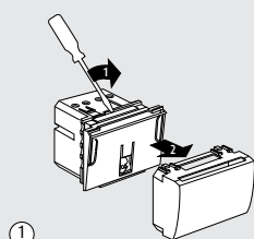
① Separar la tapa frontal del interruptor.
