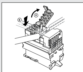
1. Abra las pestañas e inserte el cable.
