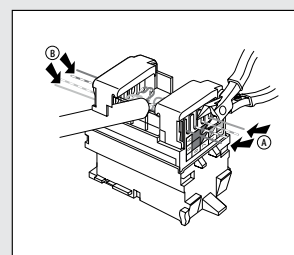
3. Corte con pinzas el cable excedente.
